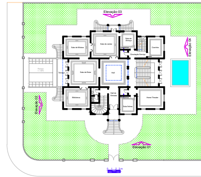
Térreo A = 260,38 m 2
